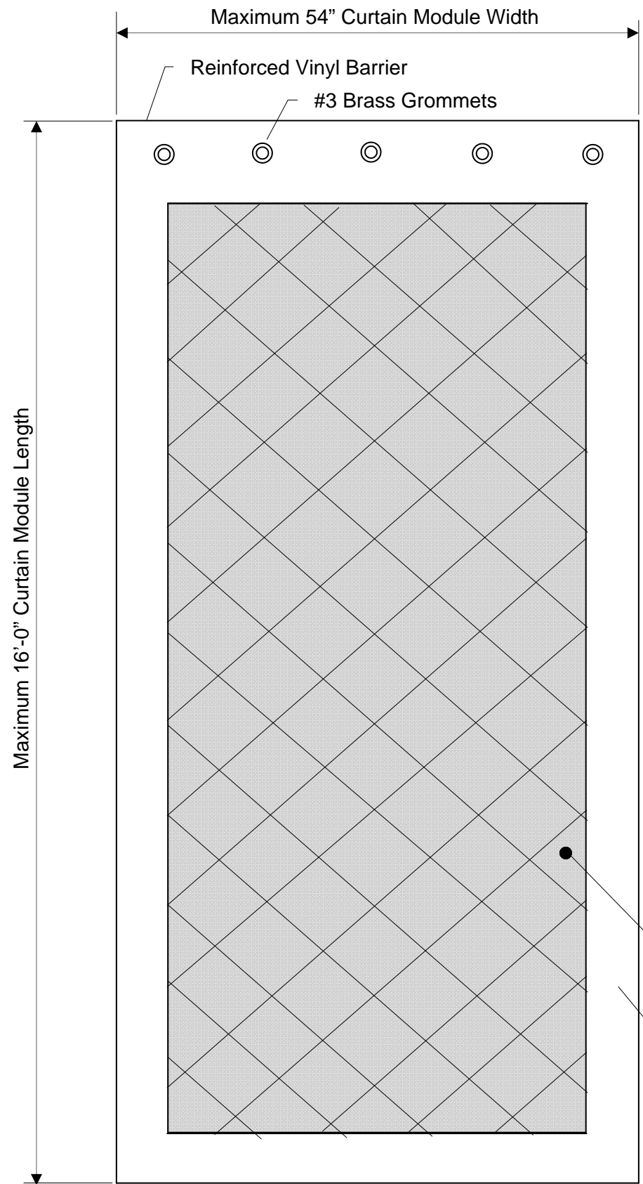
STANDARD CURTAIN MODULE
